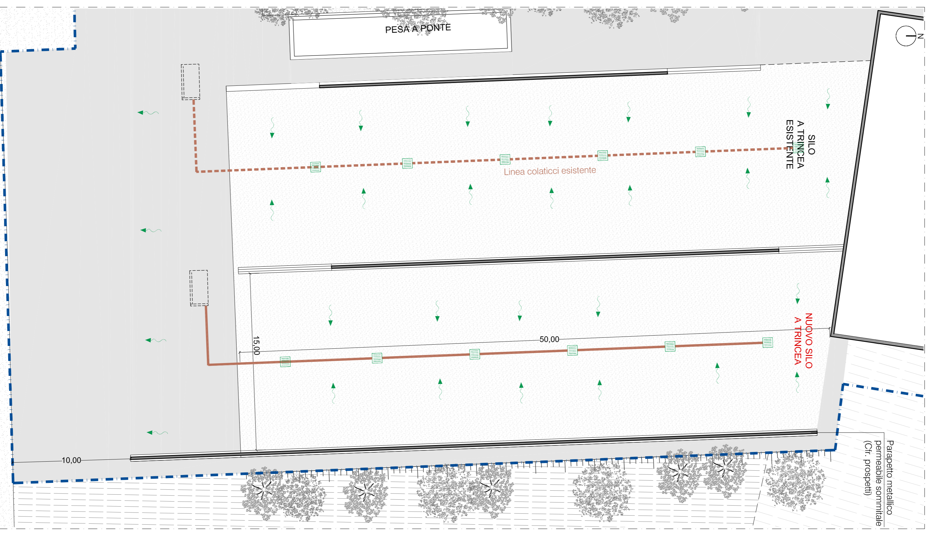
STATO DI PROGETTO - PIANTA NUOVA "TETTOIA LEGGERA" NORD - SCALA 1:200 N.B.: La tettoia è denominata "leggera" in ragione del manto di finitura scelto (telo in pvc o lamiera leggera) e pertanto è da intendersi non praticabile; quindi non necessita di dispositivi contro le cadute dall'alto
