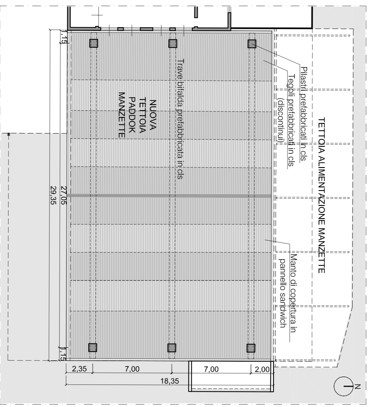
STATO DI PROGETTO - PIANTA NUOVA TETTOIA Paddock MANZETTE - SCALA 1:200
