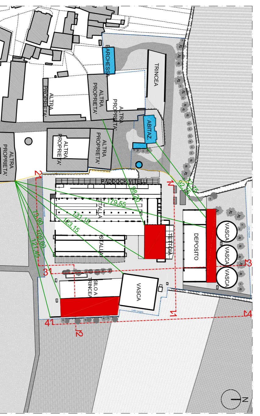
STATO DI PROGETTO - PLANIMETRIA GENERALE - SCALA 1:2000
