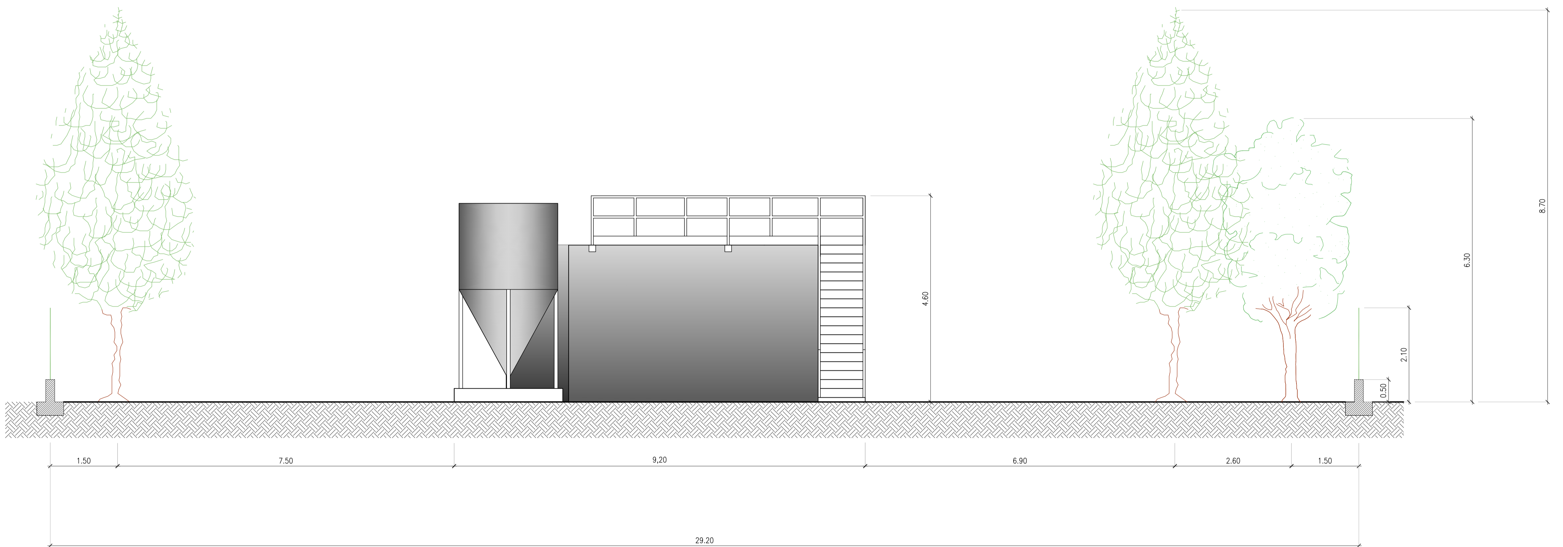
SEZIONE C-C SEZIONE SCALA 1:50
